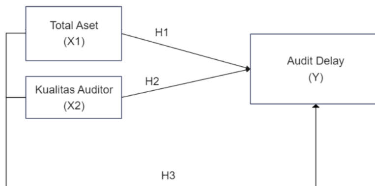
Gambar 1. Kerangka Pemikiran
